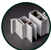
Przekrój ościeznicy RTF Standard i RTF Rewers
