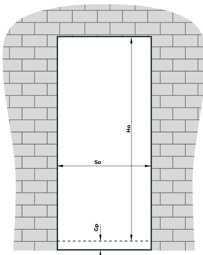
Rys.1 Wymiar otworu dla wyliczenia ościeżnicy z uwzględnieniem grubości gotowej podłogi.
