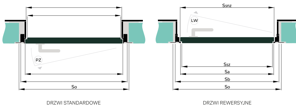
Rys.3 Przekrój poziomy przez Drzwi Standardowe i Drzwi Rewersyjne.
