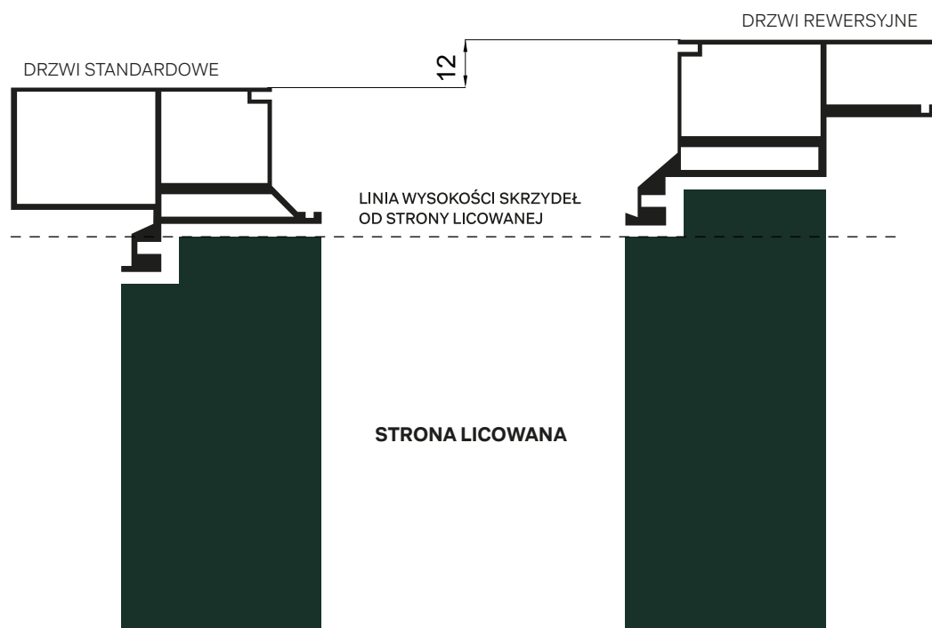
Rys.2 Różnica wysokości między Ościeżnicą Standardową a Ościeżnicą Rewersyjną przy zachowaniu takiej samej linii wysokości skrzydeł od strony licowanej.
